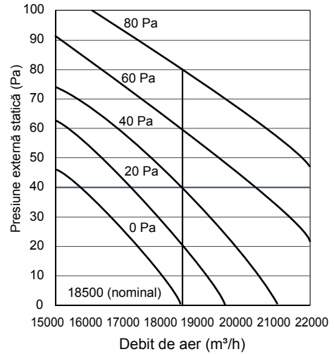
Curba de funcționare a ventilatorului 22 HP
