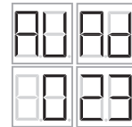
Το "AU Ad" δείχνει την αυτόματη διευθυνσιοδότηση, το "X" δείχνει τη διεύθυνση της εξωτερικής μονάδας, το "YZ" δείχνει τον αριθμό των εντοπισμένων εσωτερικών μονάδων και η παραπάνω εικόνα δείχνει τις 23 εσωτερικές μονάδες που έχουν εντοπιστεί.
