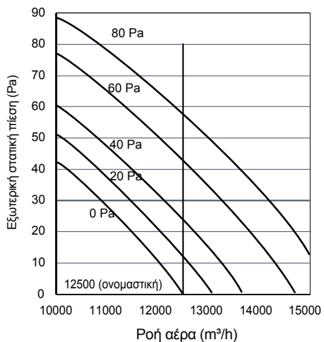
14 HP Καμπύλη χαρακτηριστικών ανεμιστήρα
