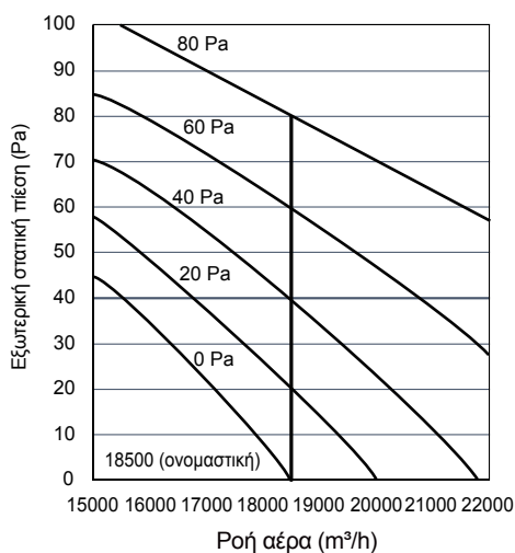
16 HP Καμπύλη χαρακτηριστικών ανεμιστήρα
