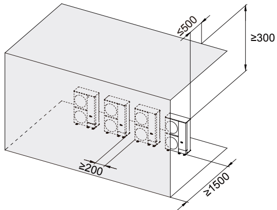
Πάνω από μία εξωτερική μονάδα Εικ. 5.8
