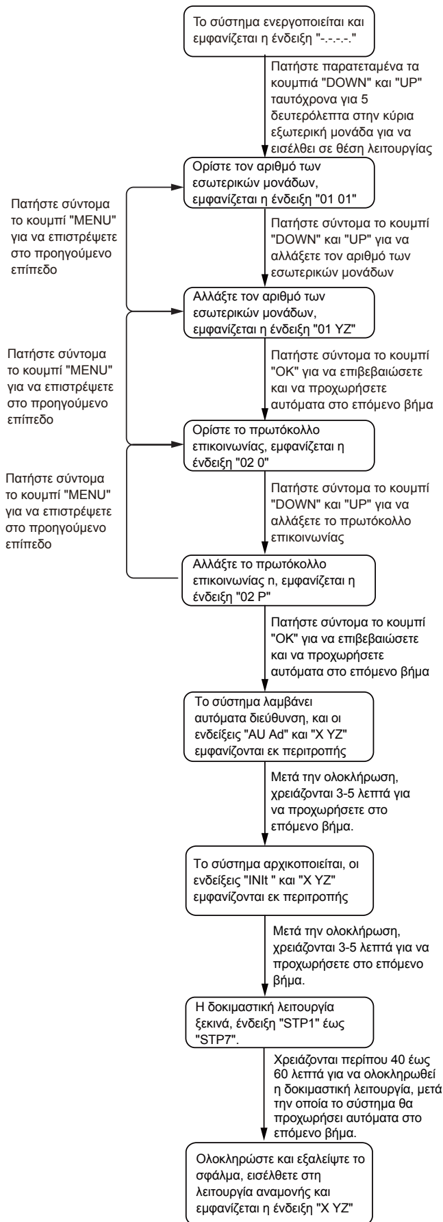
Το "STP1" αντιπροσωπεύει το βήμα 1 της δοκιμαστικής λειτουργίας ενώ το "STP7" αντιπροσωπεύει το βήμα 7.
