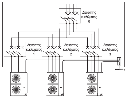
Εξωτερική μονάδα 1 Εξωτερική μονάδα 2 Εξωτερική μονάδα 3
