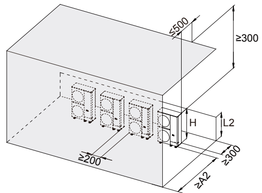
Πάνω από μία εξωτερική μονάδα Εικ. 5.10
