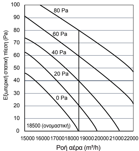
22 HP Καμπύλη χαρακτηριστικών ανεμιστήρα
