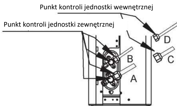
A: Zawór odcinający niskiego ciśnienia B: Zawór odcinający wysokiego ciśnienia C i D: Nakrętki kołnierzy jednostki wewnętrznej
