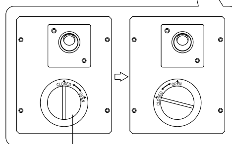
Pārbaudes vāciņš
