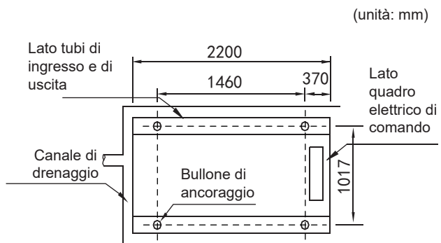
Fig. 6-6 Vista dall'alto del diagramma schematico delle dimensioni di installazione di 110 kW 140kW
