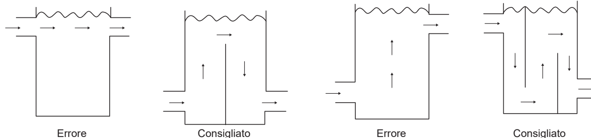
Fig. 8-20 Progettazione del serbatoio di stoccaggio
