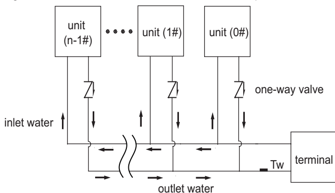
Fig. 8-24 Installazione della pompa dell'acqua multipla
