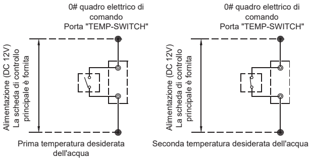
Fig. 8-14 Cablaggio della porta elettrica con campo debole "TEMP-SWITCH"
