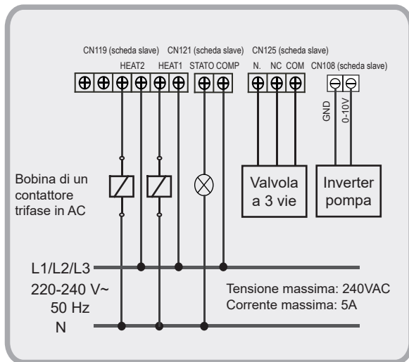
Fig. 8-11 Cablaggio del riscaldatore ausiliario della conduttura e della luce AC dello stato del compressore (50kW,65kW,75kW,110kW,140kW)
