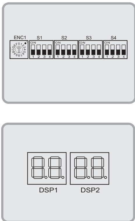
Fig. 8-7 Posizioni del display
