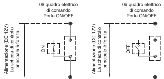
Fig. 8-12 Cablaggio della porta elettrica con campo debole "ON/OFF"
