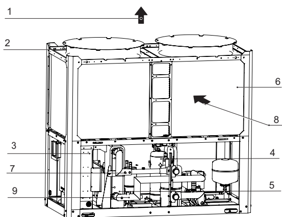
Afb. 8-1 Hoofdonderdelen van de 50KW, 50KW, 65KW, 75KW,
