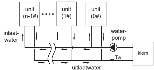
Afb. 8-24 Installatie van een enkele waterpomp
