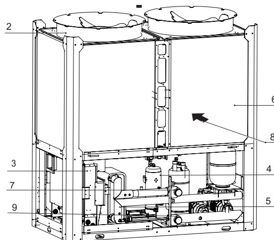
Afb. 8-2 Hoofdonderdelen van de 110KW, 140KW
