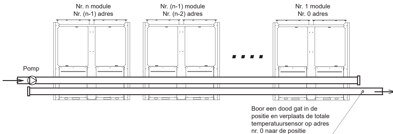
Afb. 8-22 Installatie van multimodulair systeem (niet meer dan 16 modules)
