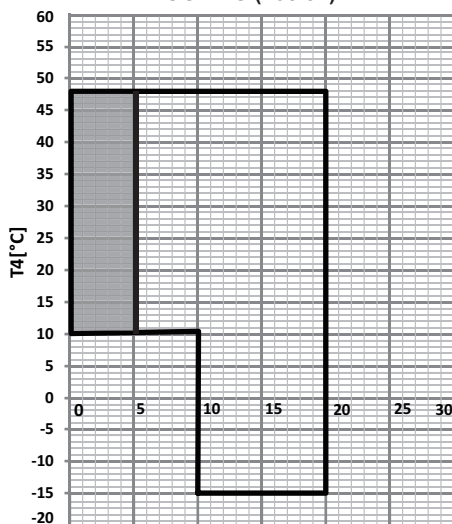
50KW, 65KW, 75KW en 110KW, 140KW COOLING (koelen)
