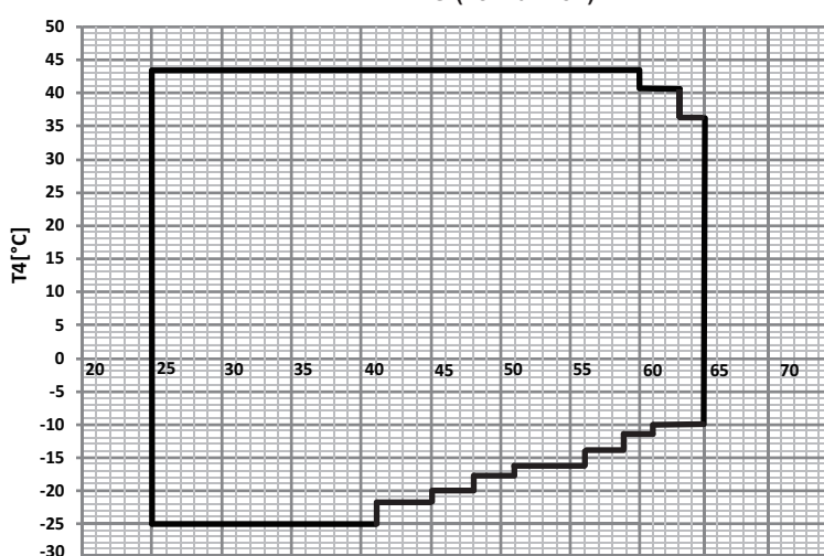
50KW, 65KW, 75KW en 110KW, 140KW HEATING (verwarmen)
