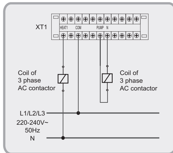
Afb. 8-20 Functie van de klemmen van de KEM-90 DNS3 KH
