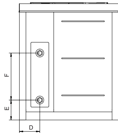
Vooraanzicht
