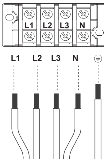
Afb 8-16 Eisen voor de aansluiting van het netsnoer
