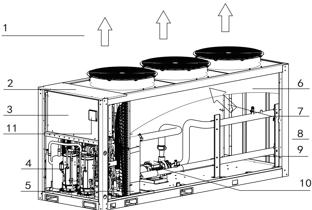
Afb. 8-3 Hoofdonderdelen van de KEM-90 DNS3 KH
