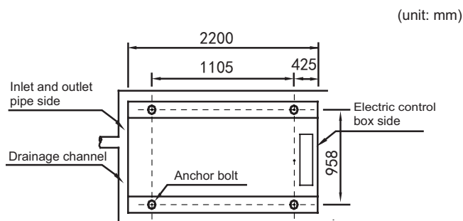
Afb. 6-8 Bovenaanzicht van het schema van de installatieafmetingen van KEM-60 DNS3 KH
