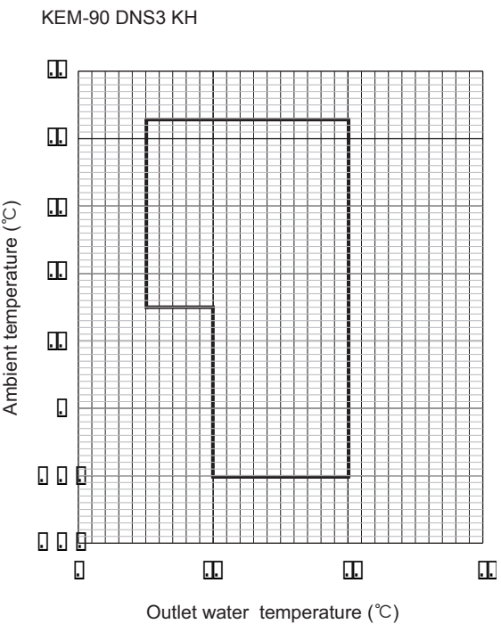
Afb. 1-2 Koelbereik van de KEM-90 DNS3 KH
