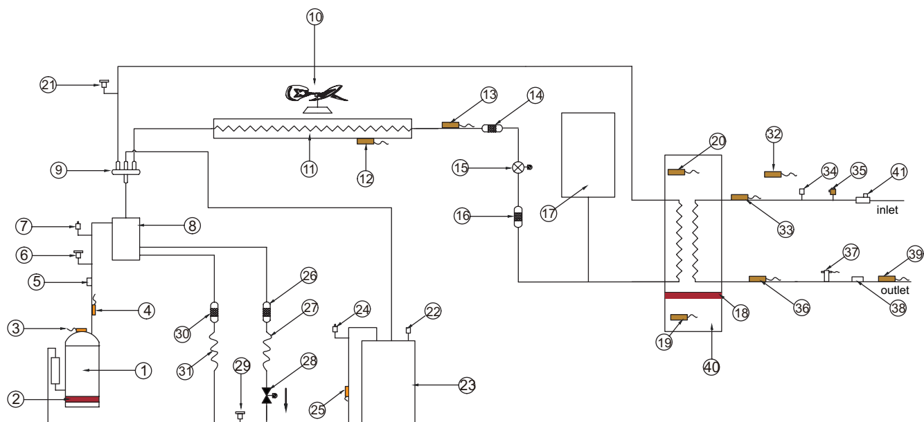
Afb. 8-7 functieschema van de KEM-30 DNS3 KH-2
