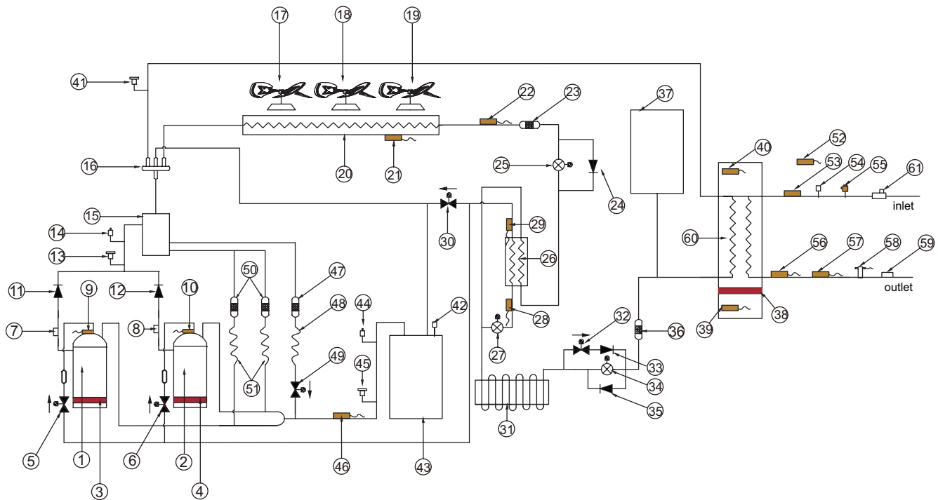
Afb. 8-9 functieschema van de KEM-90 DNS3 KH
