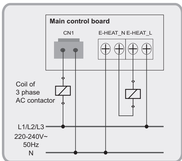
Afb. 8-19 Functie van de klemmen van de KEM-30 DNS3 KH-2 en de KEM-60 DNS3 KH
