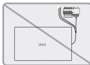
Afb. 8-24-3 Voorzorgsmaatregel besturingssysteem en installatie (c)
