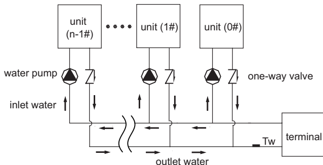
Afb. 8-36 Installatie van meerdere waterpompen
