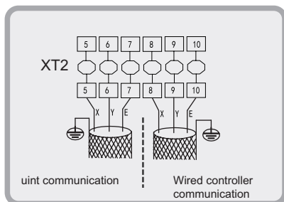
Afb. 8-18 Functie van de klemmen van de KEM-90 DNS3 KH
