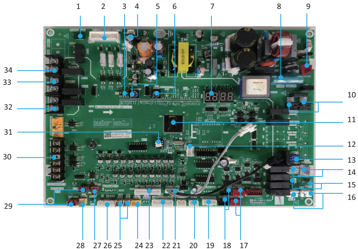
Afb. 8-10 Hoofdprintplaat van de KEM-30 DNS3 KH-2 en de KEM-60 DNS3 KH
