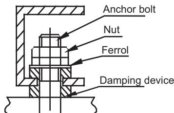
Afb. 6-10 Installatie van de demper
