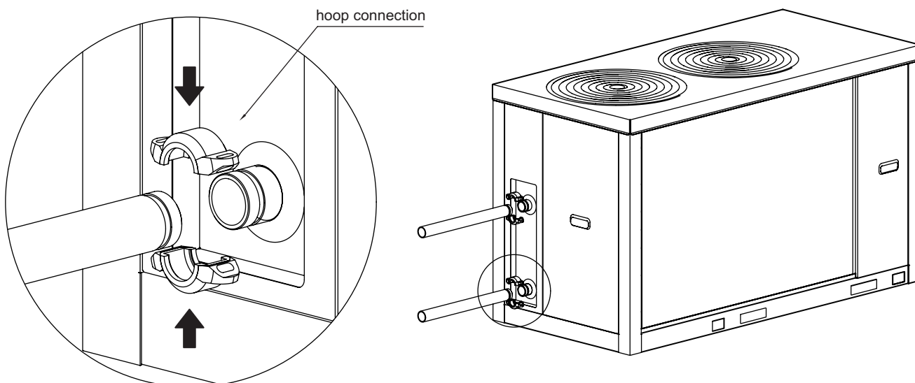
Afb. 8-29 Aansluitmethode van de leiding van de KEM-60 DNS3 KH
