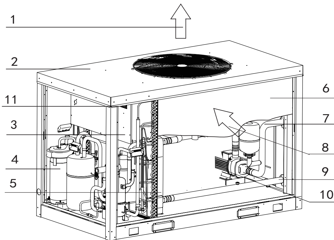
Afb. 8-1 Hoofdonderdelen van de KEM-30 DNS3 KH-2
