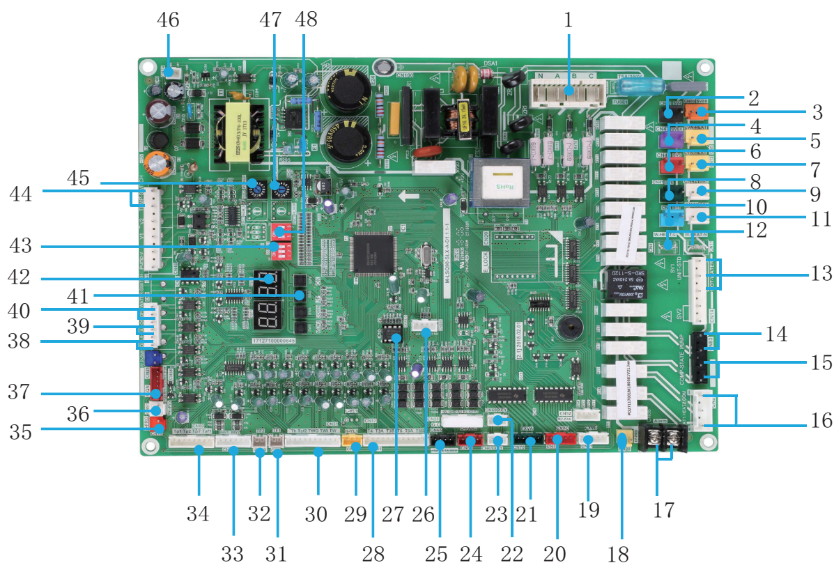
Afb. 8-11 Hoofdprintplaat van de KEM-90 DNS3 KH
