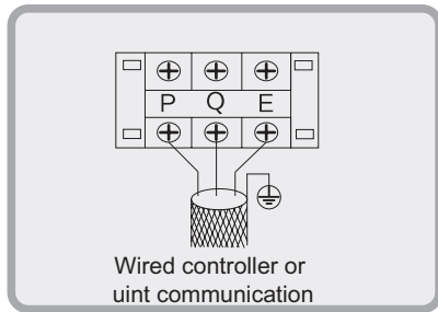
Afb. 8-17 Functie van de klemmen van de KEM-30 DNS3 KH-2 en de KEM-60 DNS3 KH
