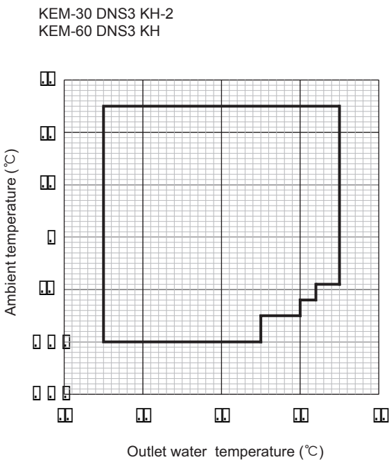
Afb. 1-3 Verwarmingsbereik van de KEM-30 DNS3 en de KEM-60 DNS3 KH
