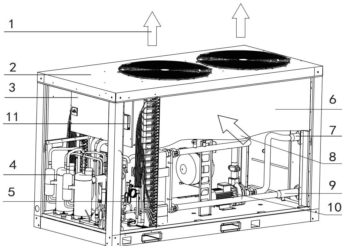
Afb. 8-2 Hoofdonderdelen van de KEM-60 DNS3 KH
