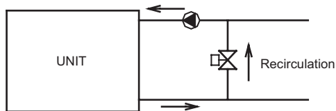
Afb. 8-32 Voor minimaal waterdebiet
