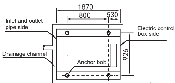
Afb. 6-7 Bovenaanzicht van het schema van de installatieafmetingen van KEM-30 DNS3 KH-2
