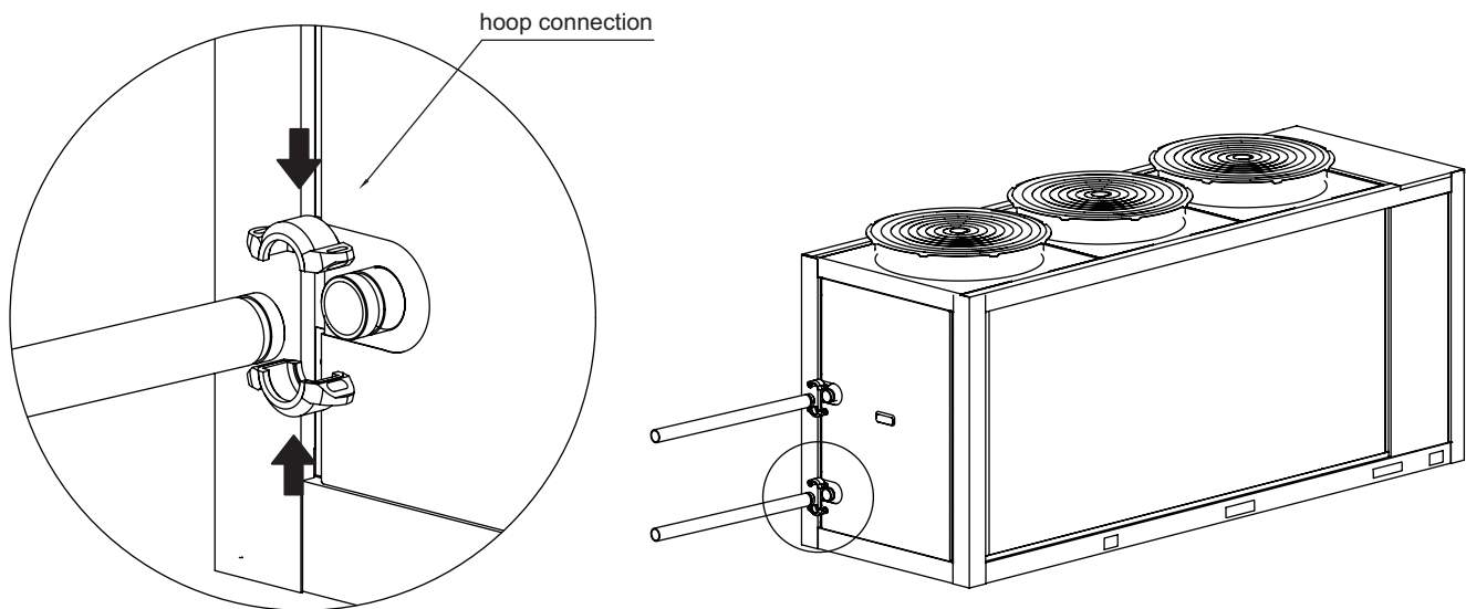
Afb. 8-30 Aansluitmethode van de leiding van de KEM-90 DNS3 KH
