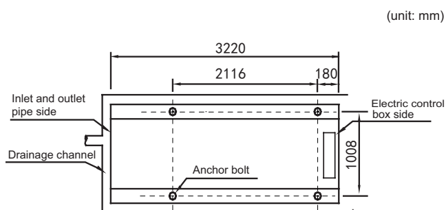
Afb. 6-9 Bovenaanzicht van het schema van de installatieafmetingen van KEM-90 DNS3 KH
