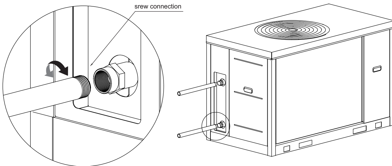
Afb. 8-28 Aansluitmethode van de leiding van de KEM-30 DNS3 KH-2
