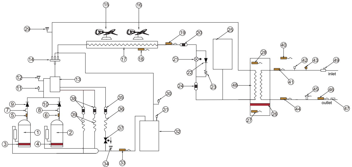
Afb. 8-8 functieschema van de KEM-60 DNS3 KH
